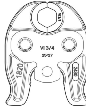
Press jaw
